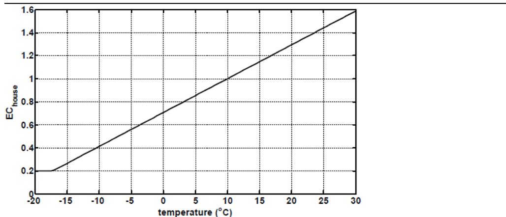
Figuur B1.4 Effect van buitentemperatuur bij profiel dierenverblijven op de emissiesterkte (EC house ; 1 is de door de gebruiker opgegeven emissiesterkte)
