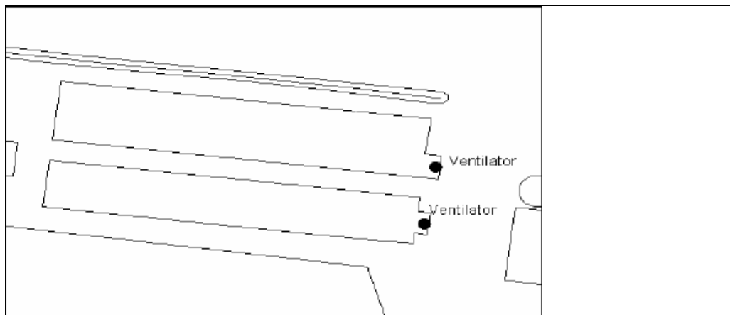
Figuur 5.1 Bepalen van de coördinaten bij centrale emissiepunten. De zwarte bolletjes zijn ventilatoren en tevens de bronnen die in AERIUS worden ingevoerd
